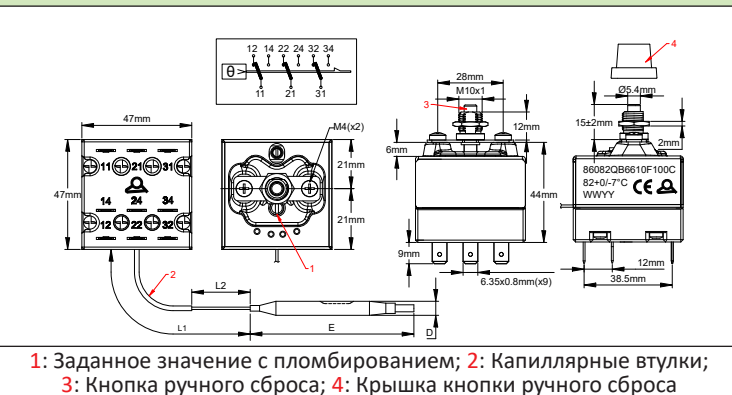
Тип с креплением при помощи центральной втулки M10
