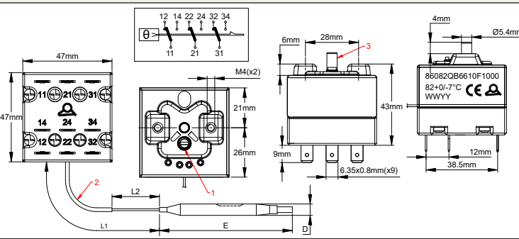
Тип с креплением 2 винтами M4
